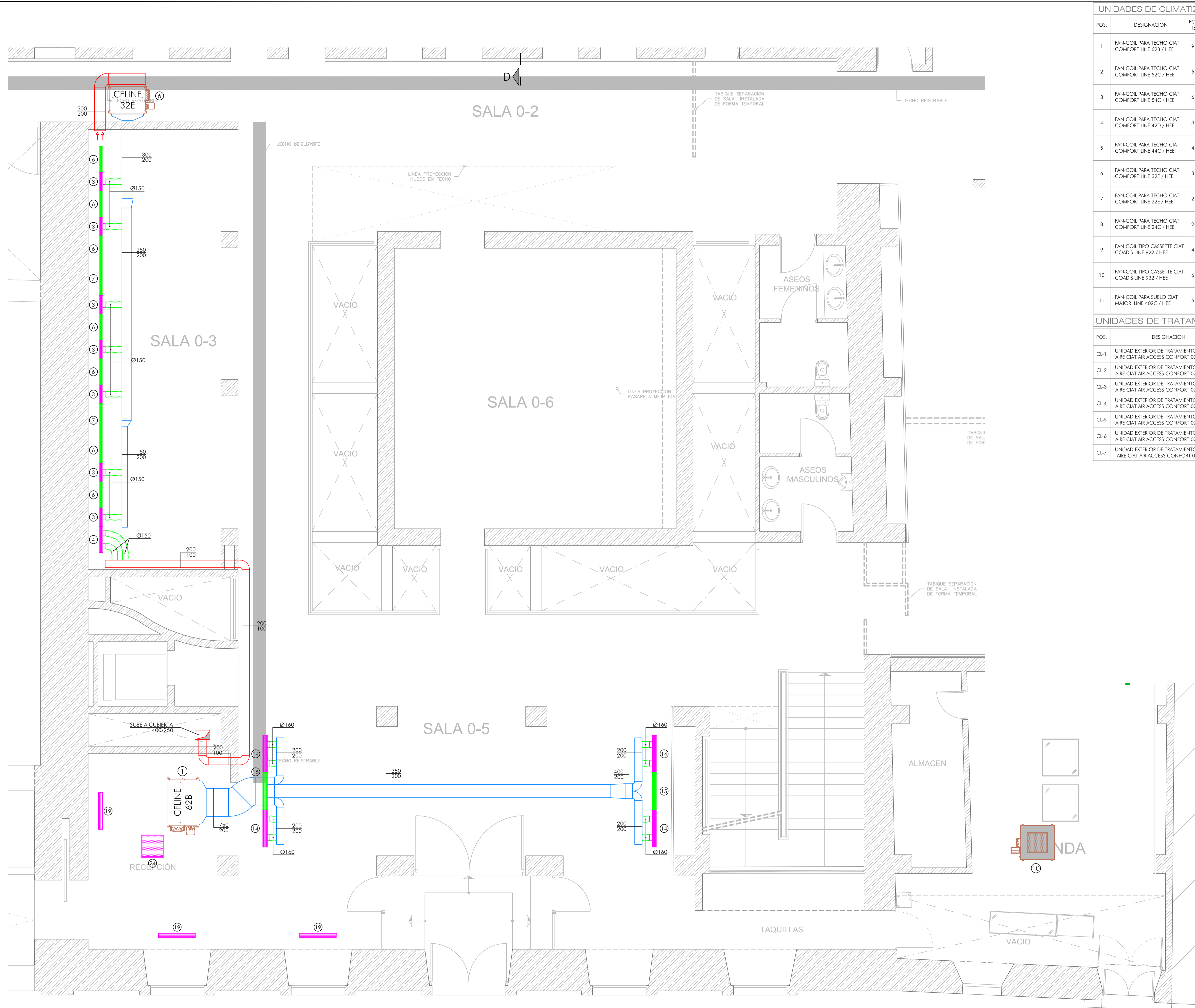
PLANTA BAJA (nivel +0.52) - RECEPCION (0-5), SALA DE EXPOSICION (0-3) Y TIENDA.
