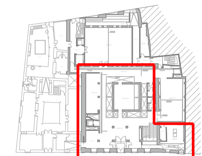
PLANTA BAJA (nivel +0.52)
