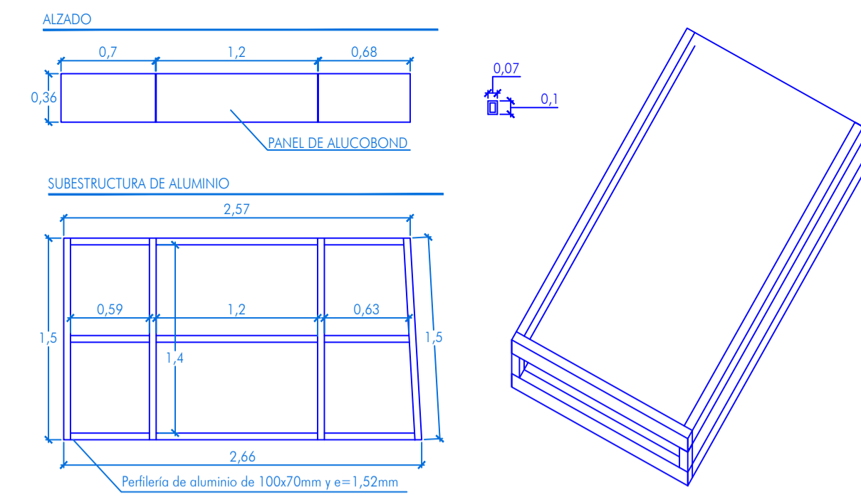
DETALLE A SUBESTRUCTURA DE ALUMINIO PARA PASO DE TUBERIAS
